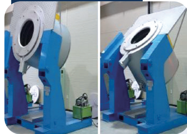
경동식 용해보온로
