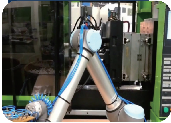
자동화 설비 로봇 (사출기)
